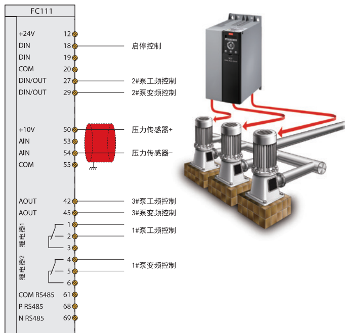
模式2：一泵两继
