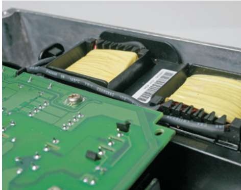
内置直流电抗器，降低谐波，延长变频器使用寿命，并节省客户外置电抗器的空间和成本
