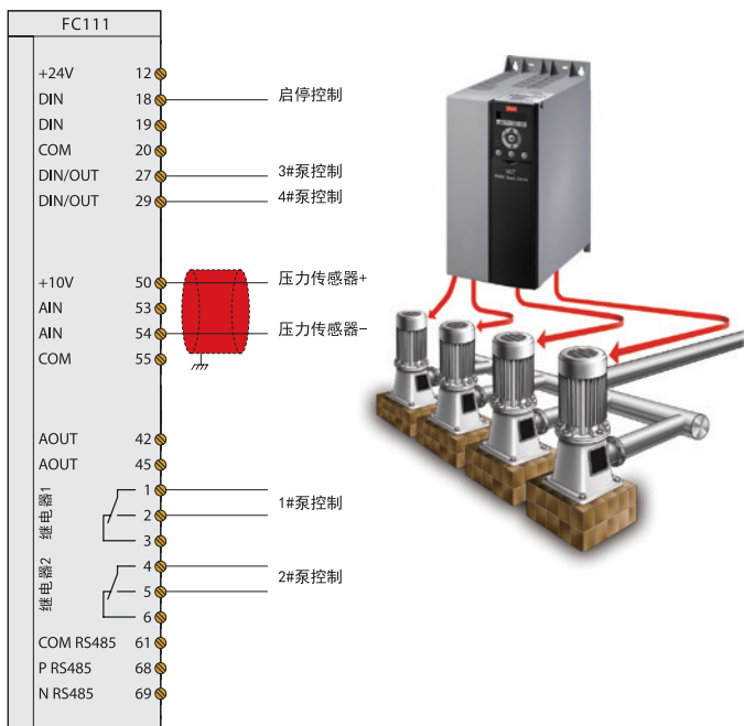
模式1：一泵一继
